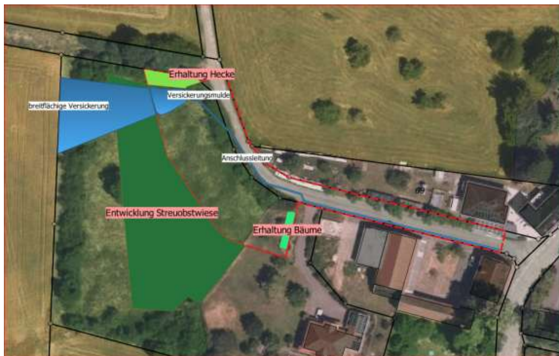
Abbildung 5: Maßnahmenplan mit externer Kompensationsmaßnahme Streuobstwiese und Versickerung Oberflächenwasser
