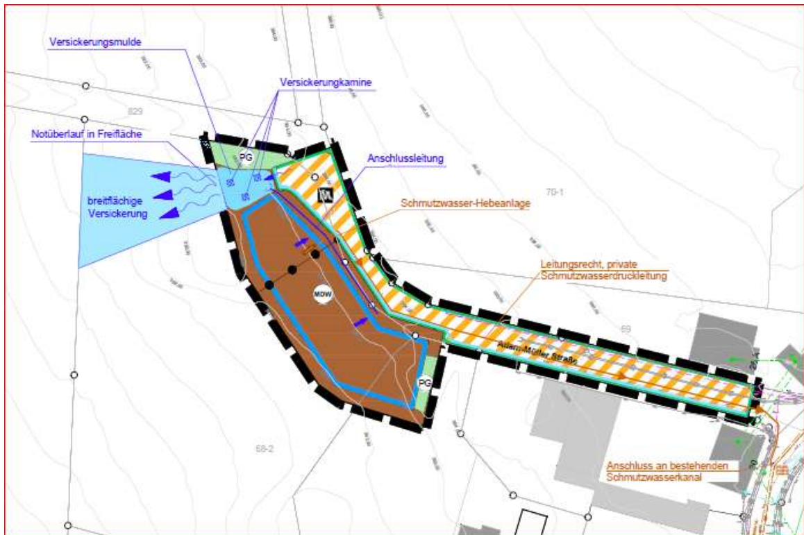
Abbildung 4: Versickerungsmulde nach Obermeyer Infrastruktur GmbH & Co. KG (2025).
