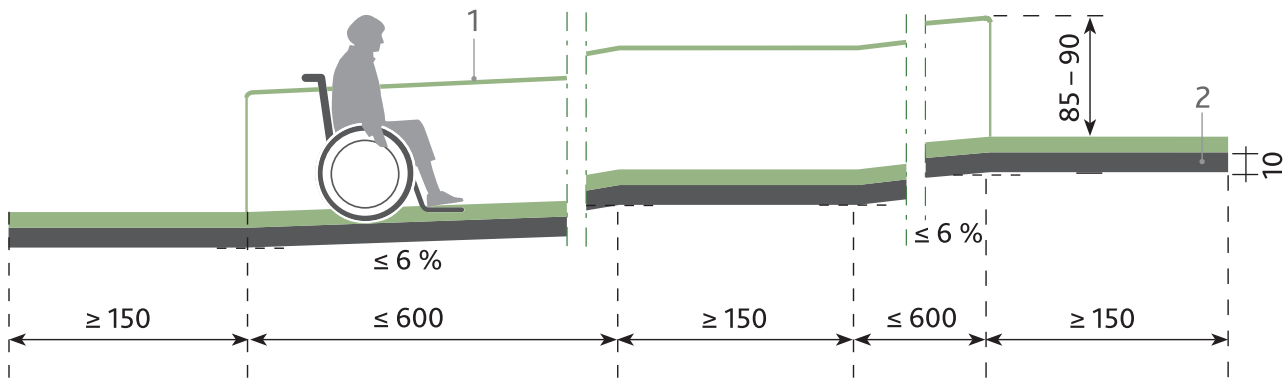
110 Seitenansicht Rampe 1 Handlauf, 2 Radabweiser
